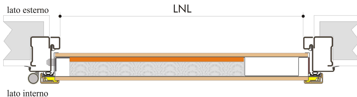
Schema rinforzi visti dall'alto
