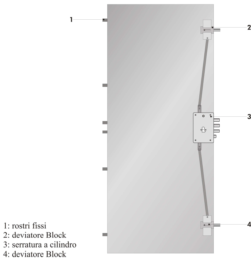
Schema sistema di chiusura
