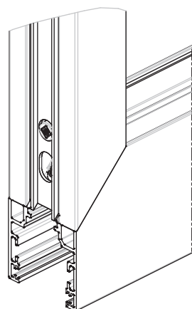
Lavorazione SX85.204 per Montaggio Tappo Copri-Lavorazione SX85.204 Machining for Cover Cap Assembly
