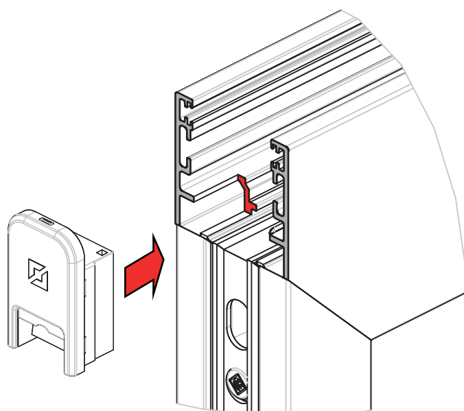
Lavorazione SX85.204 per Montaggio Tappo Copri-Lavorazione SX85.204 Machining for Cover Cap Assembly
