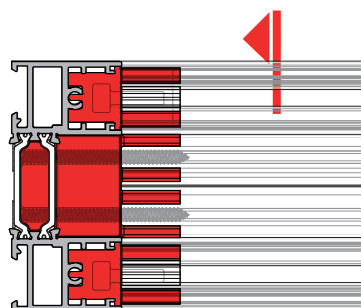
Sezione Orizzontale Horizontal Section
