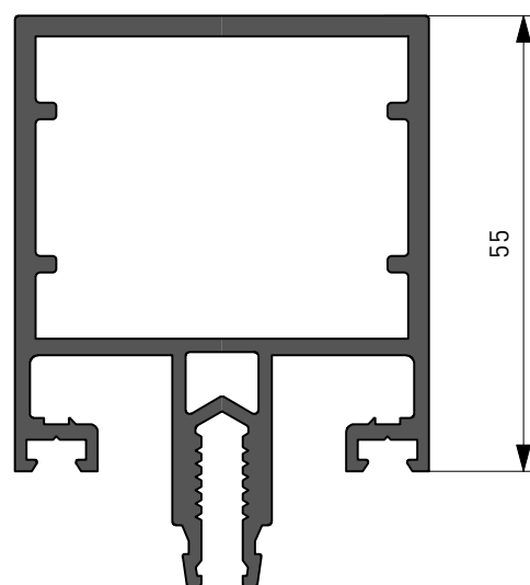
R6200 Peso 1.752 kg /ml. lxx = 26 cm4
