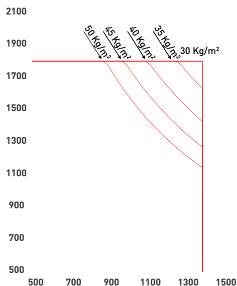
Diagramma di carico - Application range
