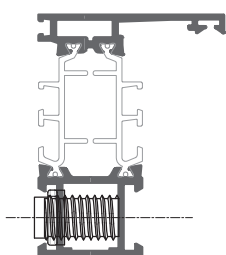
ARX.06.02 Piastrina registro Telaio Plate adjusting screw
