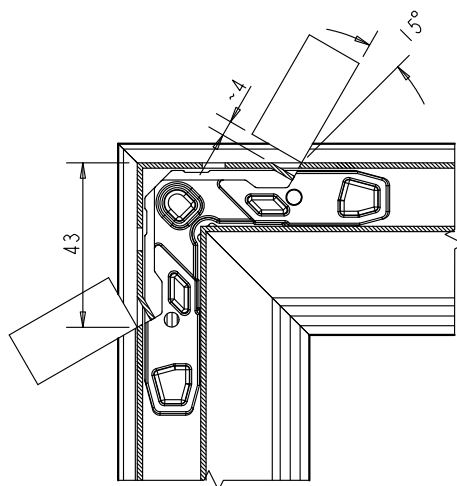
CIANFRINATURA Coltello 10 mm RIVETING Knife 10 mm
