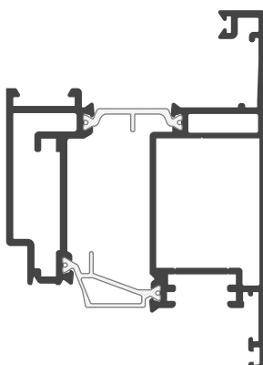
ACX.03.72 Movimentazione Bidirezionale Interasse 23 - 35 mm Bi-directional movement Center Distance 23 - 35 mm
