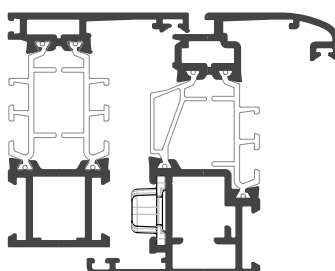
ACX.08.13 Incontro Asta singolo in ZAMA Single Zamac Bar Rest Plate
