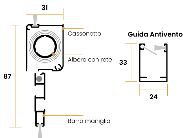
Sezione orizzontale
